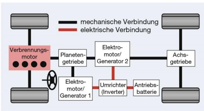
Abb.5: Gemischter Hybridantrieb (Schema)
