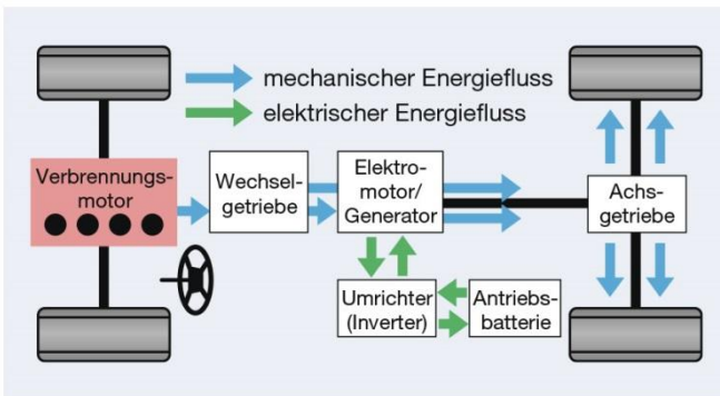
Abb.4: Paralleler Hybridantrieb (Schema)
