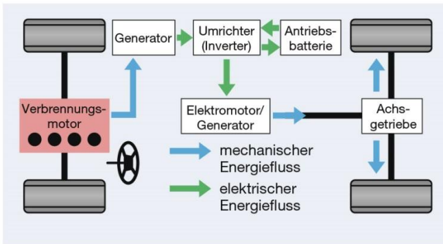
Abb.3: Serieller Hybridantrieb (Schema)
